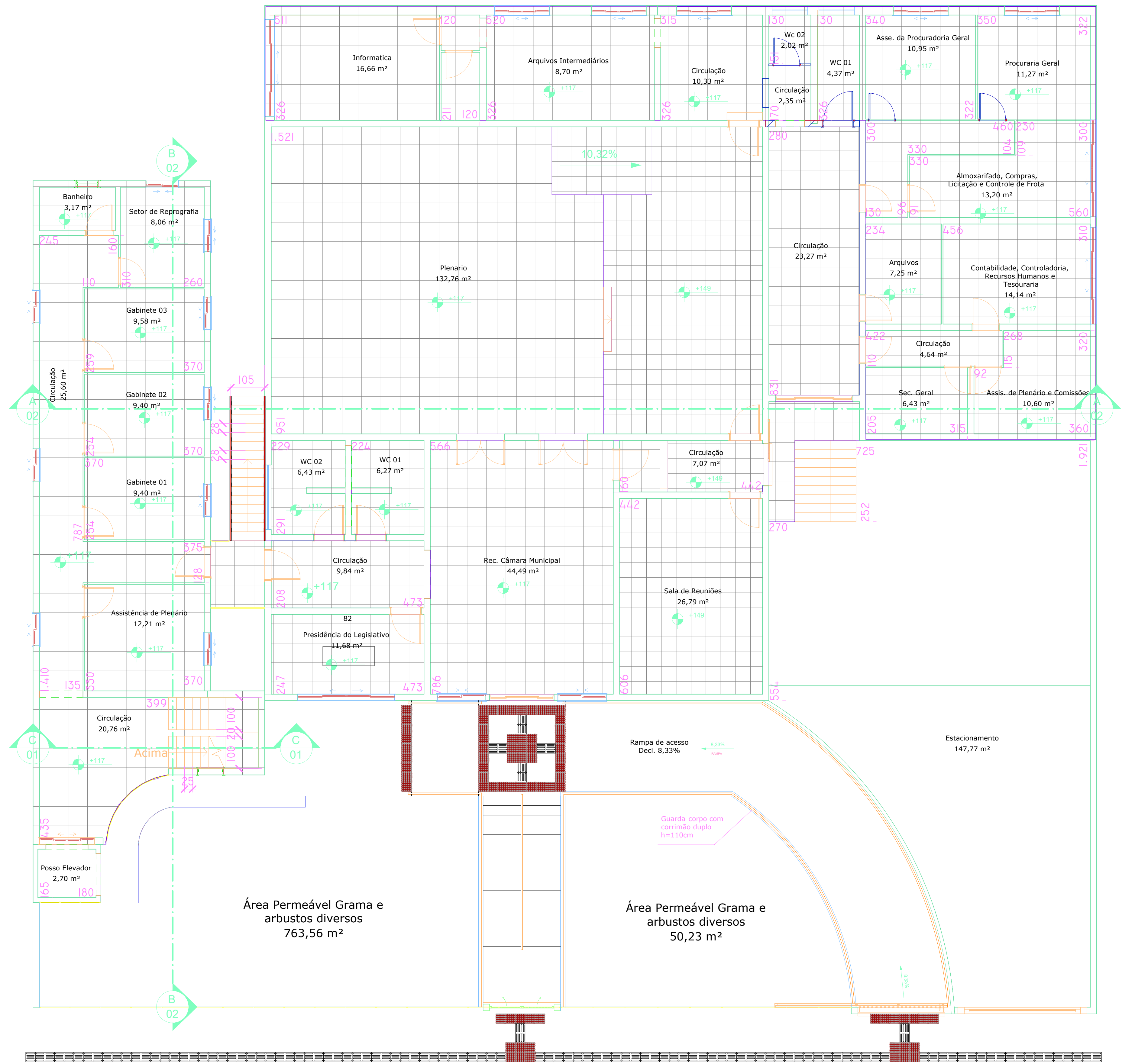
2 Térreo ESCALA 1 : 100
