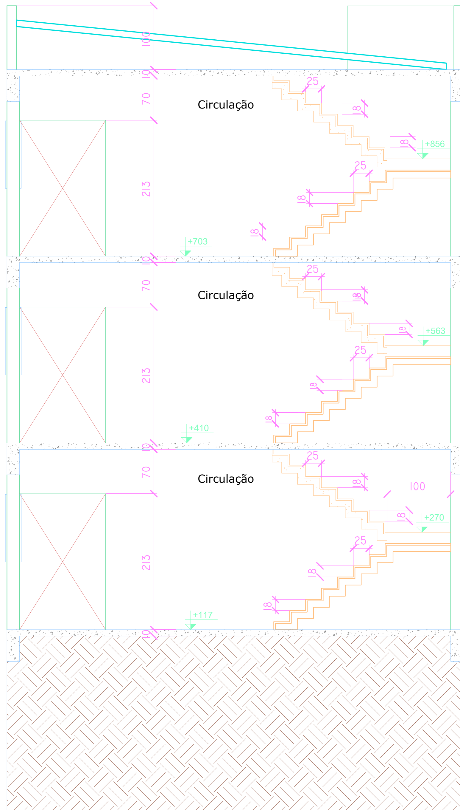
4 Corte C-C ESCALA 1 : 50
